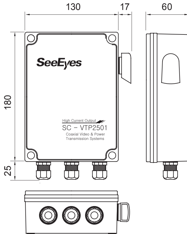
送信機(SC-VTP2501)
