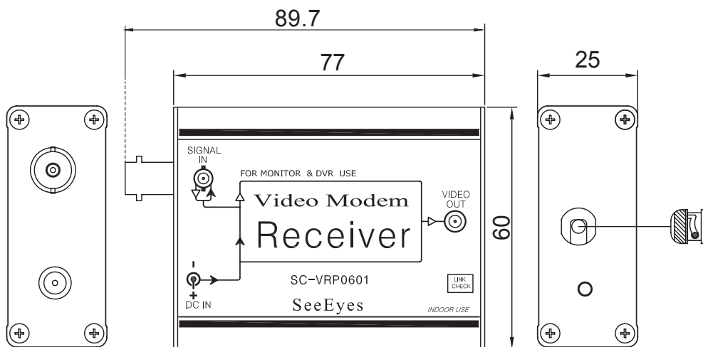
受信機(SC-VRP0601)
